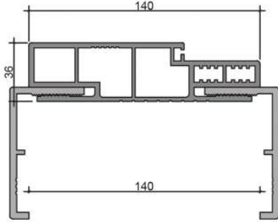
14 CM KASA 85*45 PERVAZ
