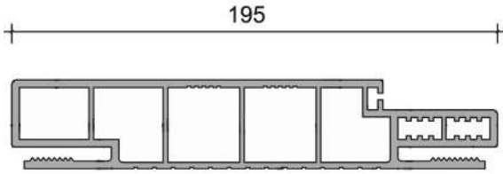
195 mm KASA 195 mm FRAME
