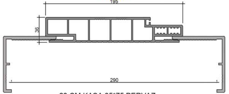
20 CM KASA 85*75 PERVAZ
